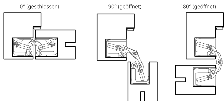
180° Öffnungsbereich des TECTUS-Drehtürbandes
